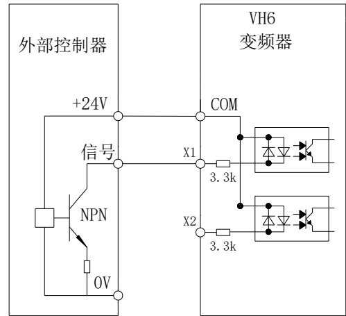
使用外部24V电源的漏型接线方法
